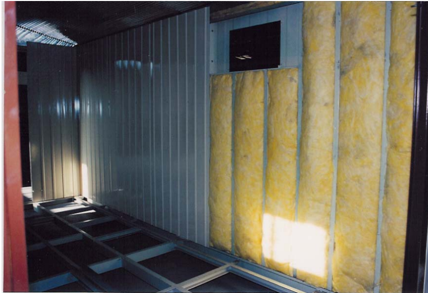
İKİNCİ ETAP İzolasyonun üzerinin galvaniz saca kapatılması
